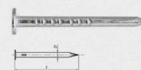
Гвозди толевые
