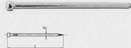
Гвозди финишные
